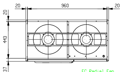
EC Radial Fan
