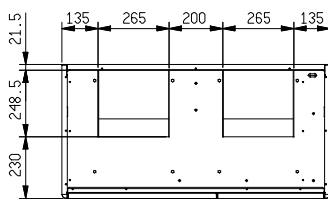
Centrifugal Fan
